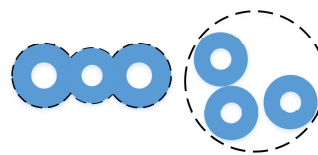
Fig. 2. Sección transversal de un cable multipolar plano (izquierda) y un cable monopolar (derecha) de tres conductores. Nótese que en el caso del cable monopolar, la distancia entre los conductores varía a lo largo de la línea ya que estos van sueltos dentro de una estructura rígida, típicamente un tubo de plástico corrugado
